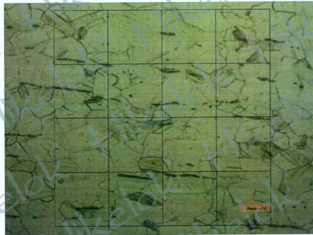
1661325-1-1 视场 5 200X 1661325-1-1 field5 200X
